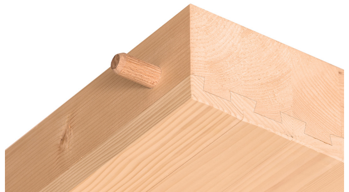
Schwalbenschwanzverbindung
